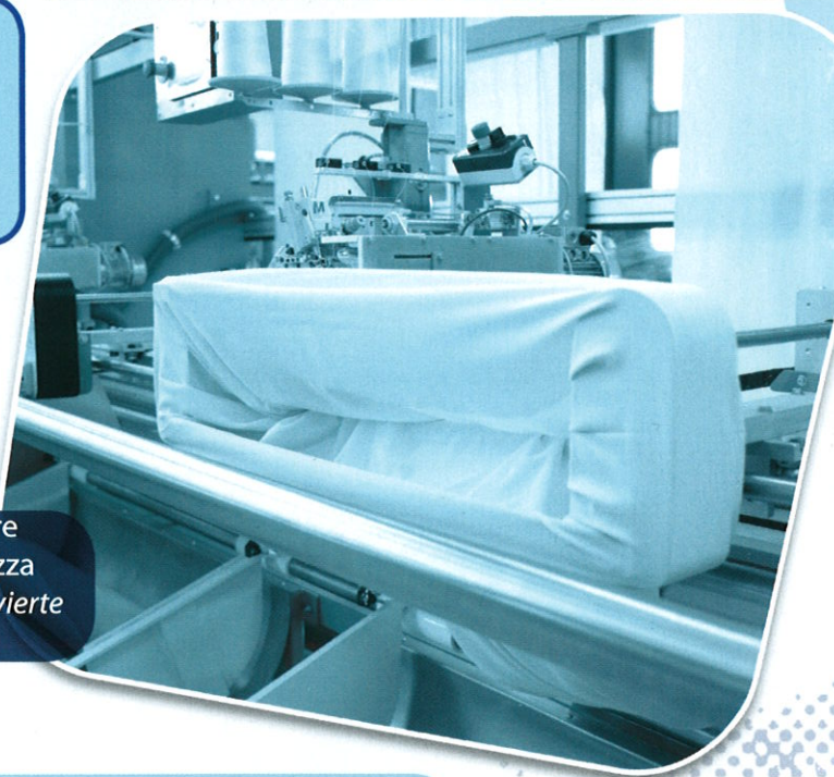
Portatessuto in cucitura a mezzo 2 nastri motorizzati a posizione variabile in funzio- ne del diametro del tubolare
